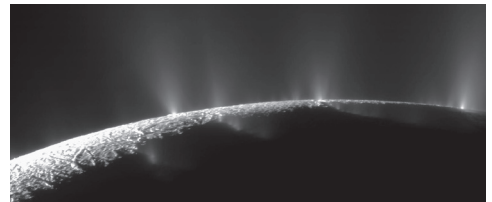
Enceladus Jets
