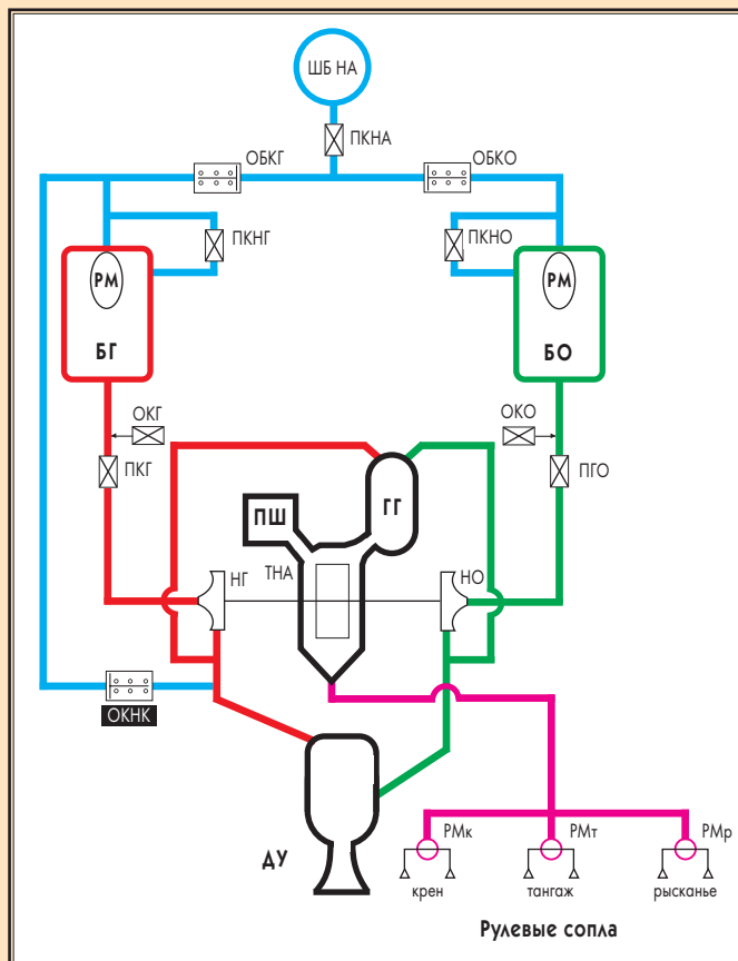
Рис. 2. Пневмогидросхема ТДУ
