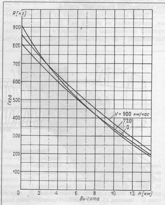
Высотная характеристика двигателя
