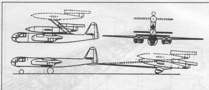
Схемы самолета Ar-234C в вариантах носителя и буксировщика самолетов-снарядов Fi-103
