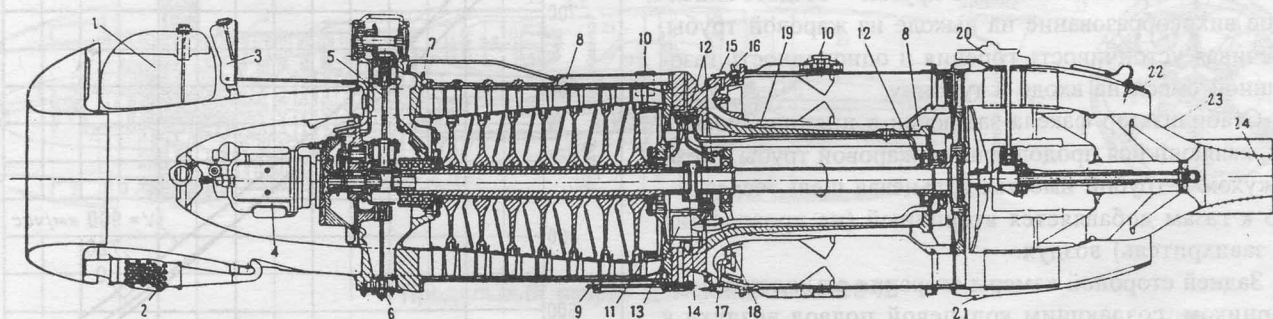
Турбореактивный двигатель BMW-003
