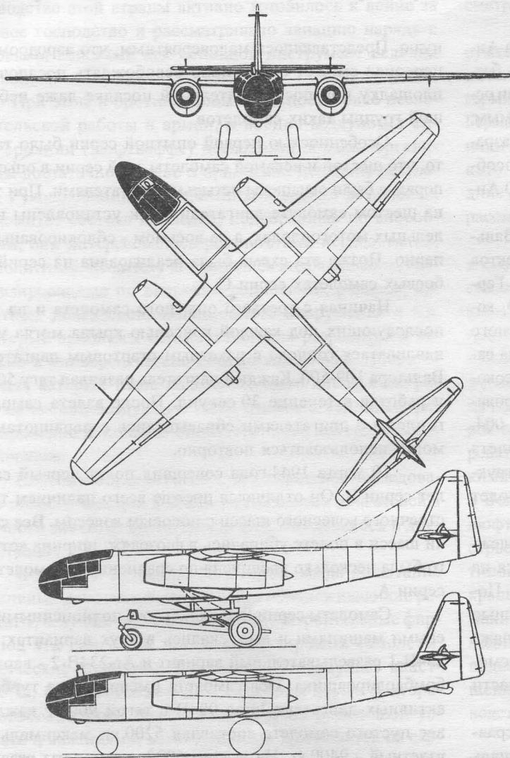
Схемы реактивного бомбардировщика Ar-234B-2 и опытного самолета Ar-234A
