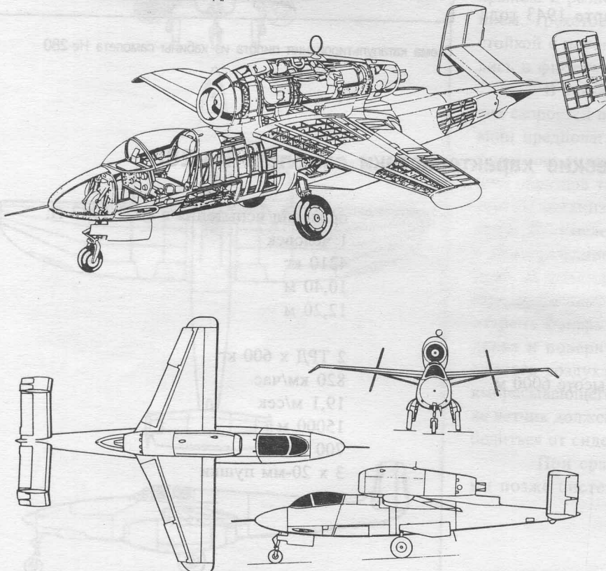
Компоновочная схема и проекции истребителя He-162A-2 “Саламандра”
