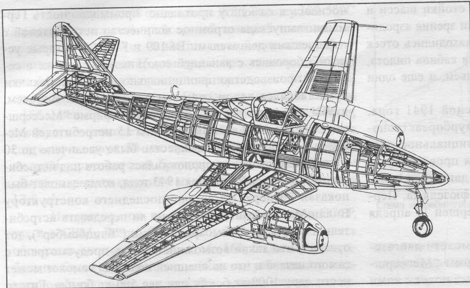
Компоновочная схема реактивного истребителя Me-262A-1a "Швальбе"
