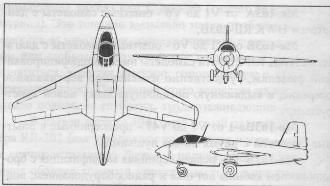
Схема истребителя-перехватчика Me-263
