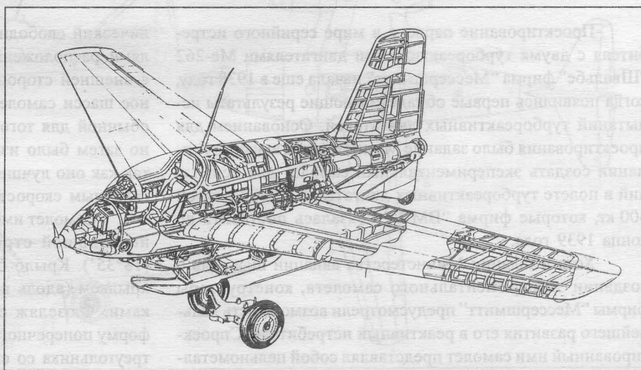
Компоновочная схема истребителя Me-163B-1a “Комета”
