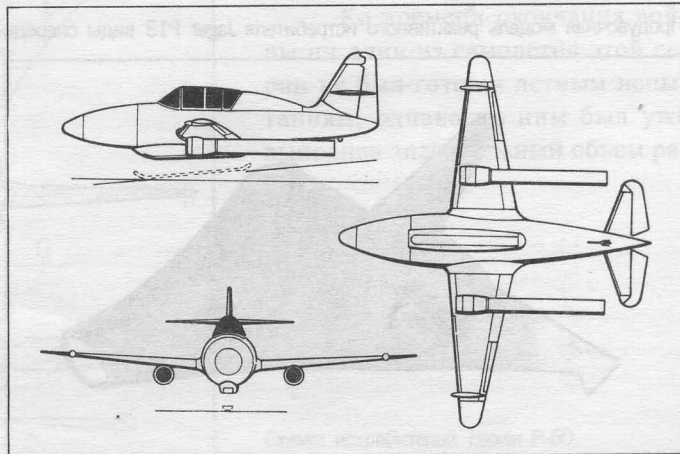
Схема реактивного штурмовика Me-328B
