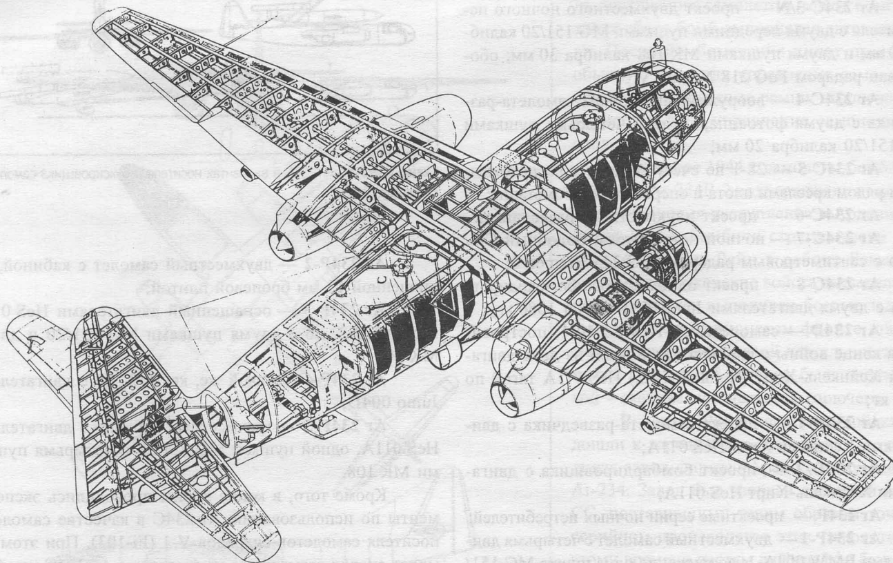
Компоновочная схема самолета Ar-234 "Блиц"
