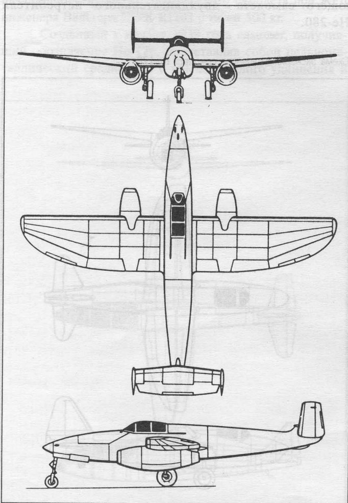
Схема истребителя He-280
