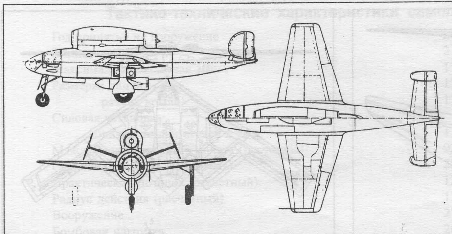
Схема пикирующего бомбардировщика Hs-132
