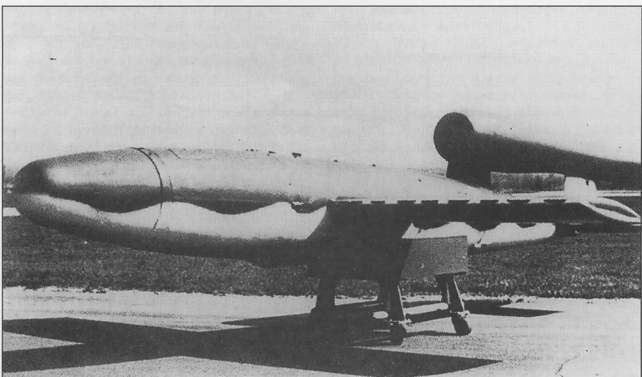
Опытный экземпляр самолета-снаряда FZG 76 на транспортной тележке. Снимок сделан на полигоне в Пенемюнде.
