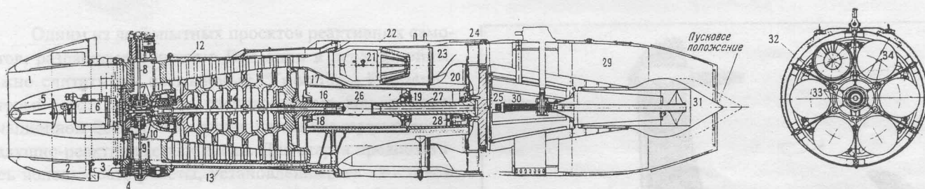
Продольный разрез двигателя Jumo-004В
