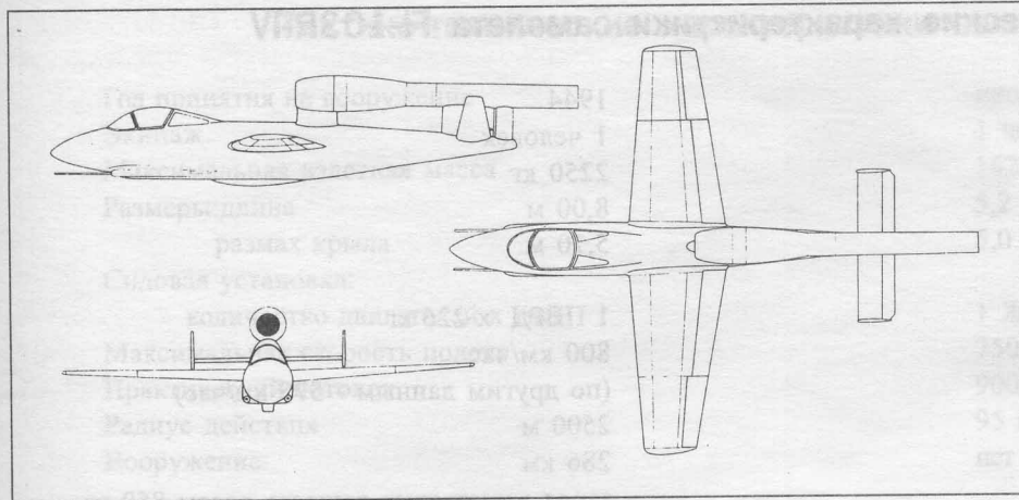
Схема легкого штурмовика EF-126, разработавшегося в 1946 году ОКБ-1 в Дессау по заданию советской администрации
