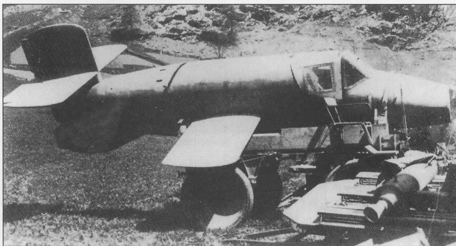
Один из экземпляров самолета «Наттер», захваченный американскими войсками в апреле 1945 года на заводе в Вальдзее. Самолет находится на транспортной тележке, в правом нижнем углу снимка виден стартовый пороховой двигатель «Шмиддинг».
