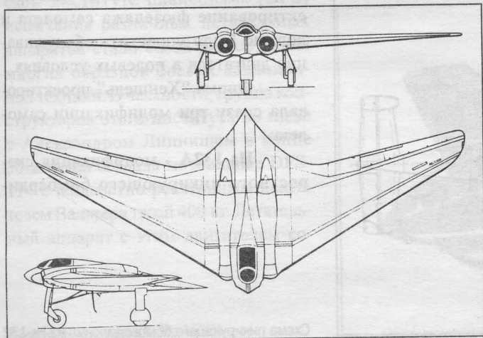
Схема истребителя-бомбардировщика Go-229
