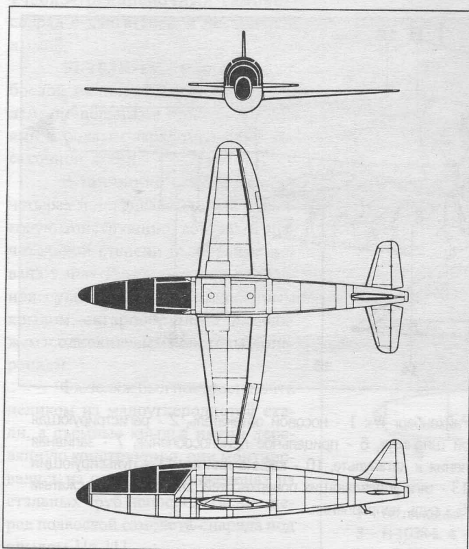
Схема экспериментального самолета He-176
