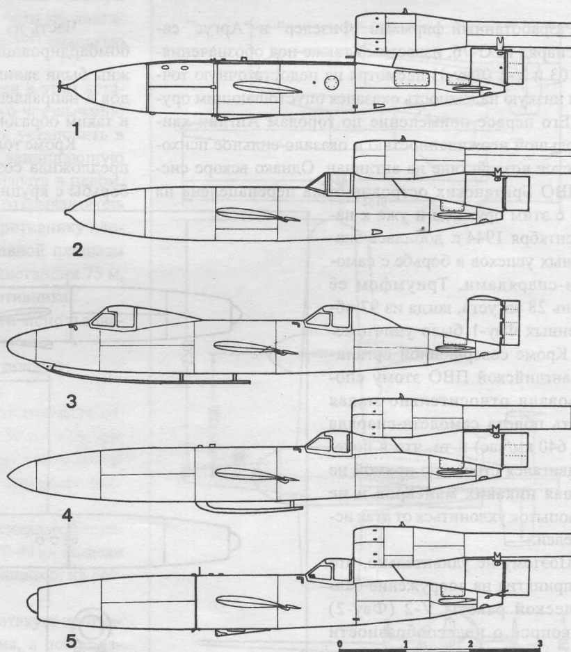
Немецкие самолеты-снаряды времен второй мировой войны
