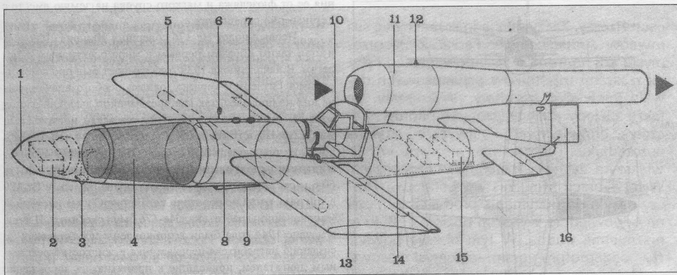
Конструктивная схема пилотируемого самолета-снаряда «Райхенберг IV»: 1 - носовой обтекатель, 2 - регистрирующая аппаратура, 3 - взрыватель, 4 - боевая часть, 5 - трубчатый силовой шпангоут, 6 - прицельное приспособление, 7 - заливная горловина топливного бака, 8 - топливный бак, 9 - устройство крепления к катапульте, 10 - кабина пилота, 11 - пульсирующий воздушно-реактивный двигатель Argus As-014, 12 - запальная свеча, 13 - тяги управляющих поверхностей, 14 - баллон со сжатым воздухом для двигателя, 15 - аппаратура управления двигателем, 16 - руль направления.
