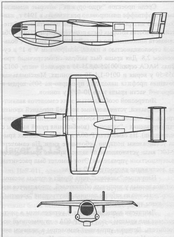
Схема истребителя-перехватчика Р.1077 "Юлия"
