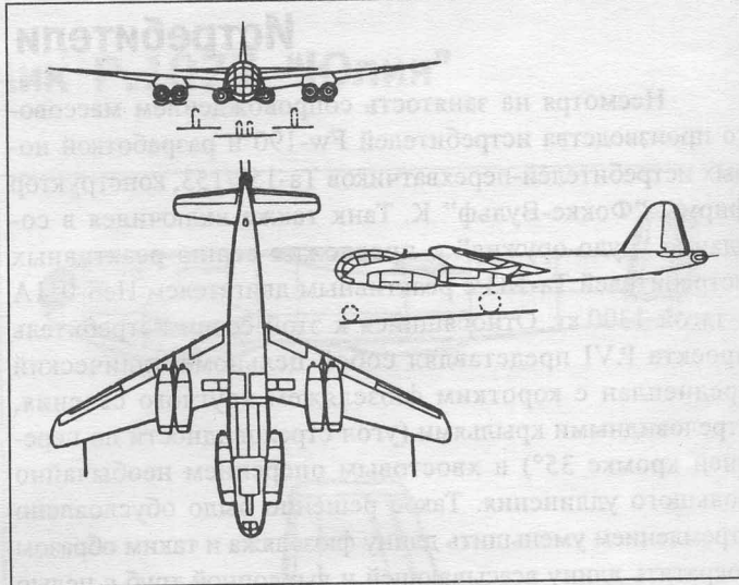
Тяжелый бомбардировщик Ju-287V-3 с шестью реактивными двигателями
