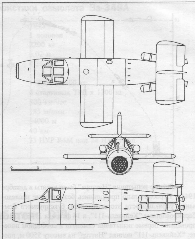
Схема истребителя-перехватчика Ва-349В-1
