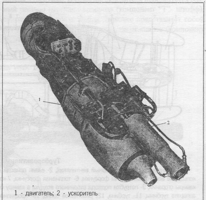
Турбореактивный двигатель BMW-003 с жидкостным ускорителем
