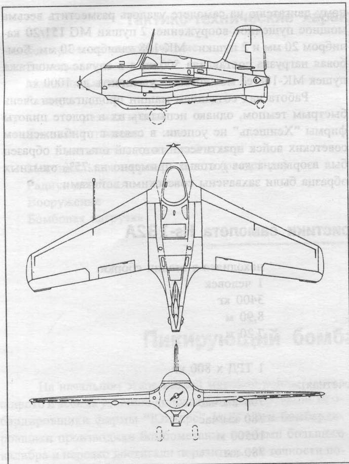
Схема ракетного истребителя Me-163
