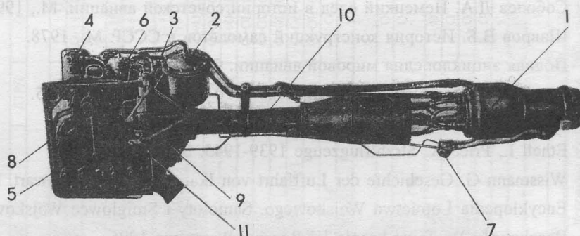
Общий вид двигателя HWK-109-509
