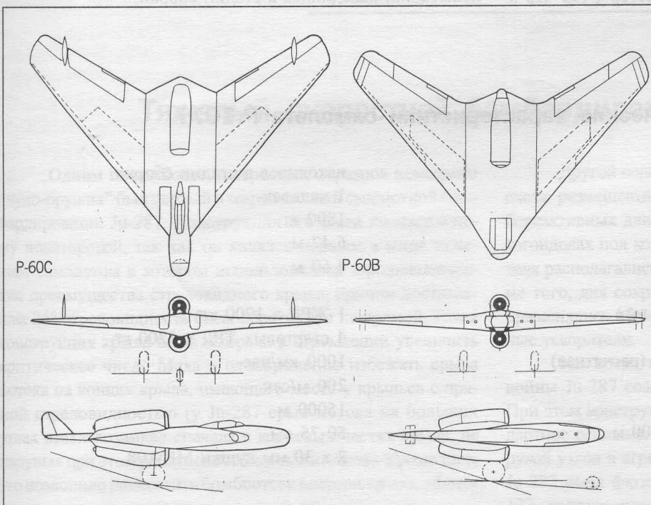
Схемы истребителей серии P-60
