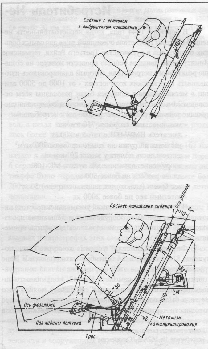
Схема катапультирования пилота из кабины самолета He-280
