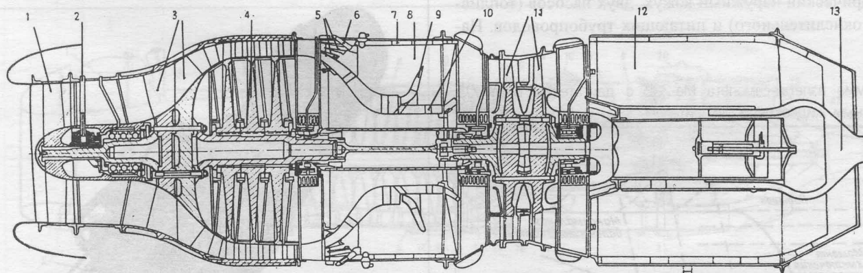
Турбореактивный двигатель HeS-011
