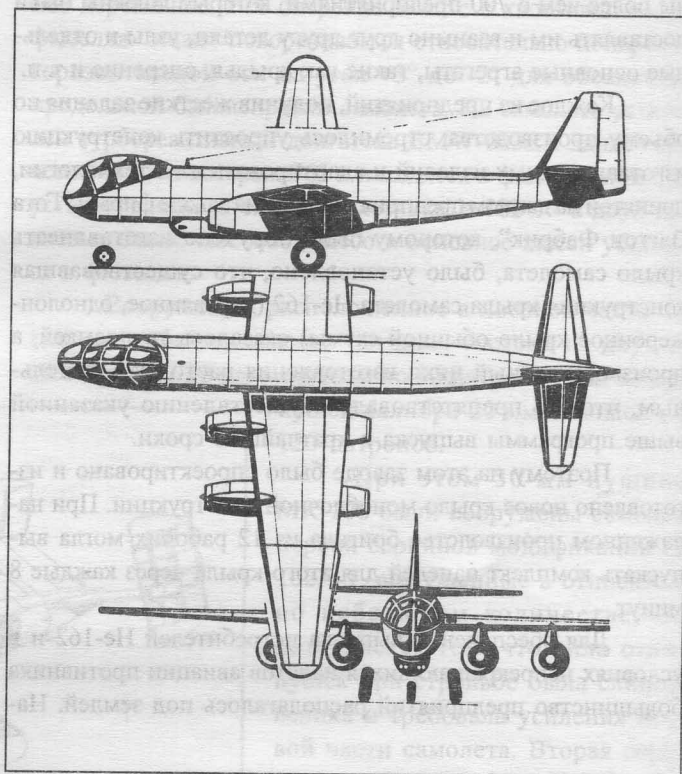
Схема бомбардировщика He-343
