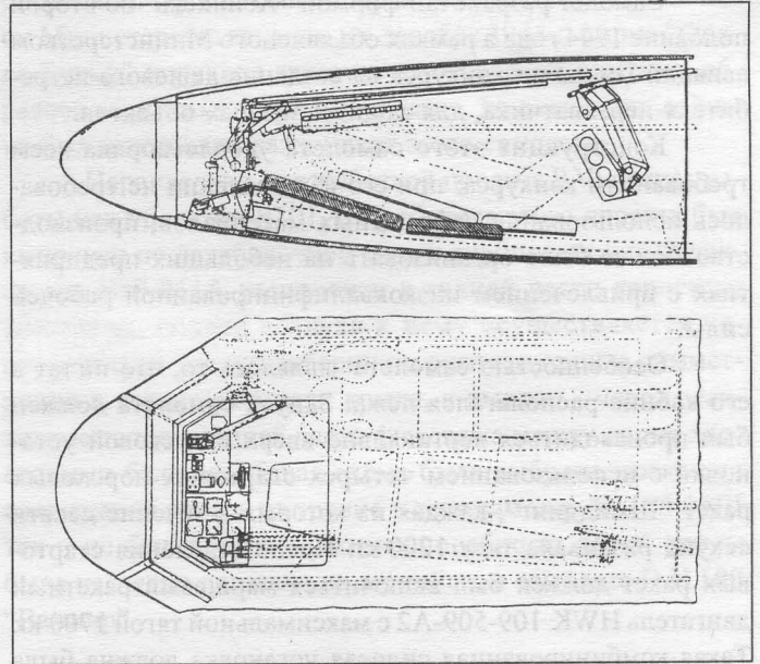
Схема расположения экипажа в кабине истребителей P-60A и P-60B
