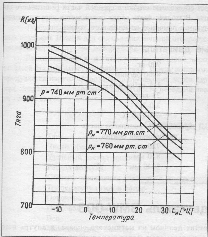
Изменение тяги двигателя в зависимости от температуры и давления атмосферного воздуха
