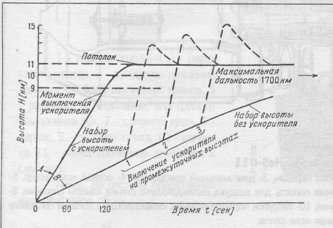
Барограмма взлета самолета Me-262 с двигателем BMW-003, снабженным жидкостным ускорителем
