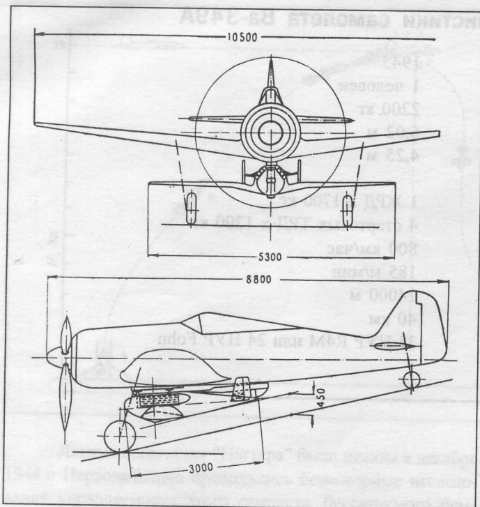
Истребитель Fw-190 с подвешенным под ним планером-истребителем
