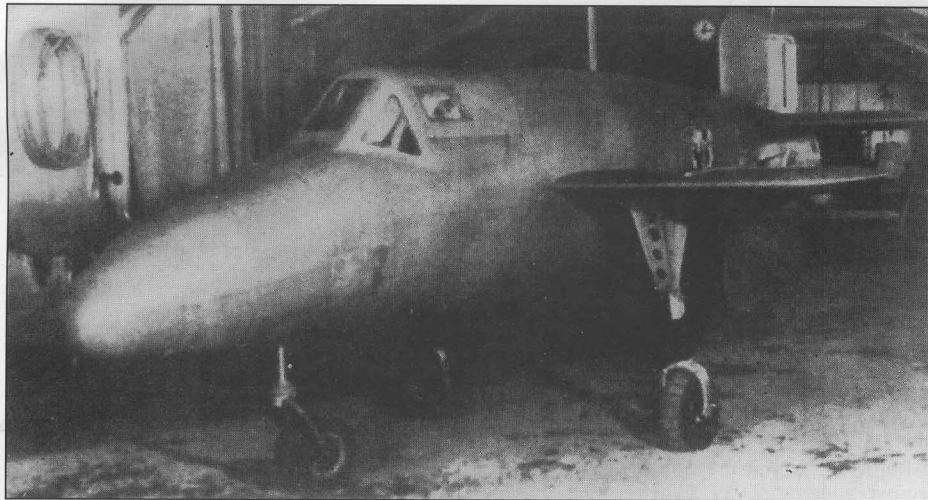
Готовый к летным испытаниям макет самолета Ва-349А. Снимок сделан в помещении заводского цеха в феврале 1945 года.
