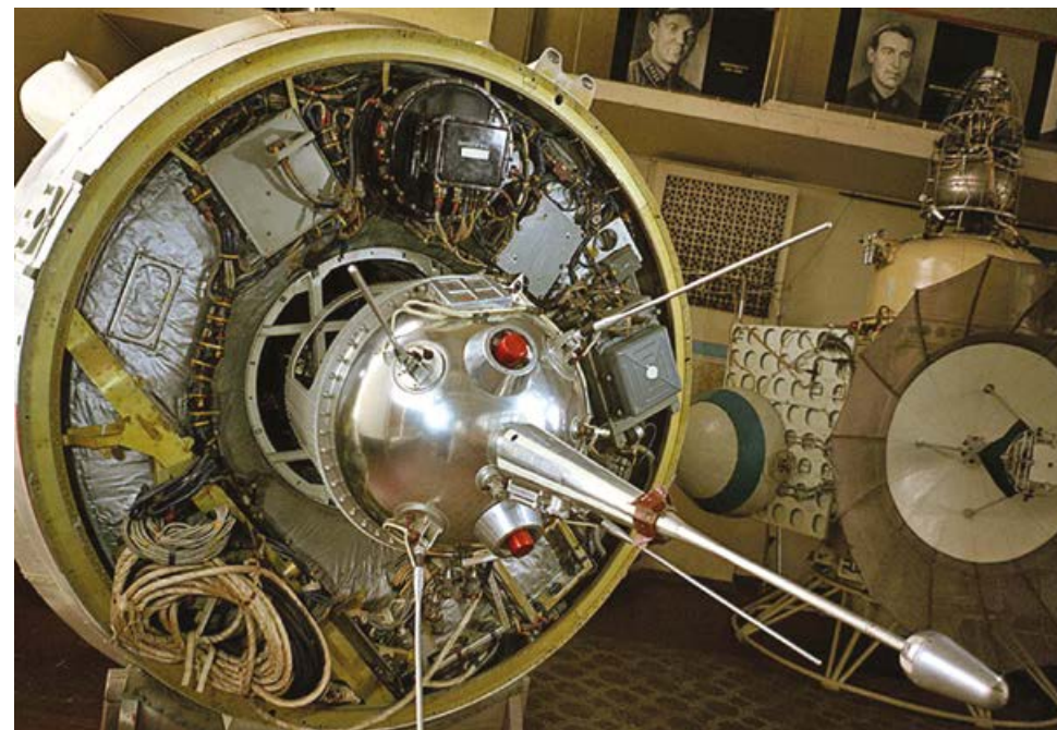
Автоматическая межпланетная станция «Луна-2» – первая в мире станция, достигшая поверхности Луны в сентябре 1959 г.
